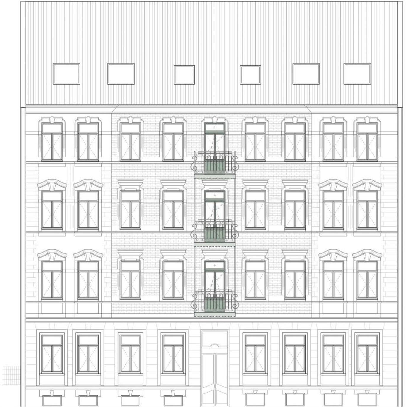
STRASSENANSICHT, FASSADE
